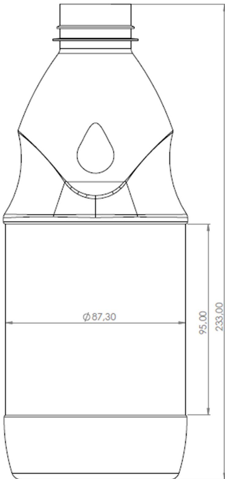
Anexo I – Desenho Técnico
