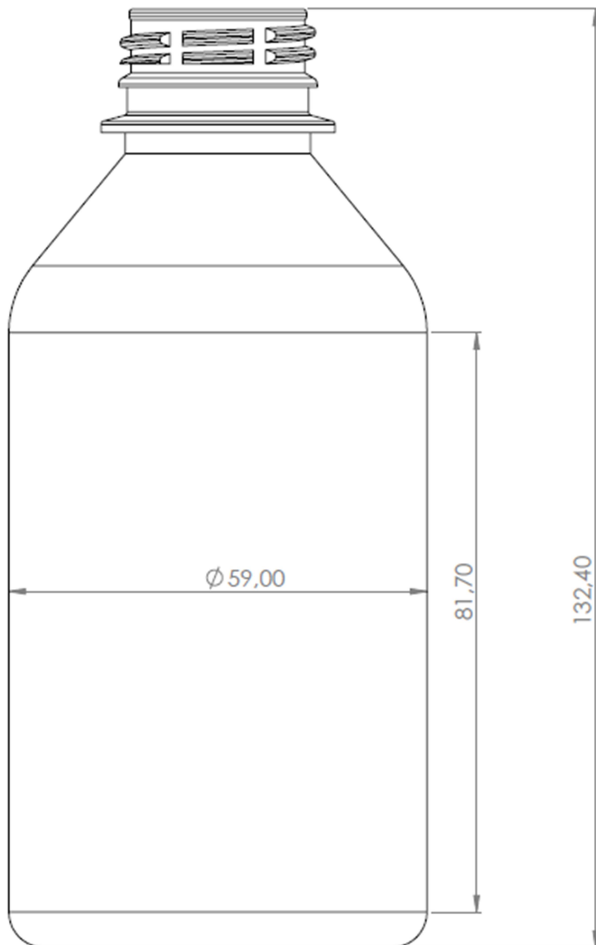
Anexo I – Desenho Técnico
